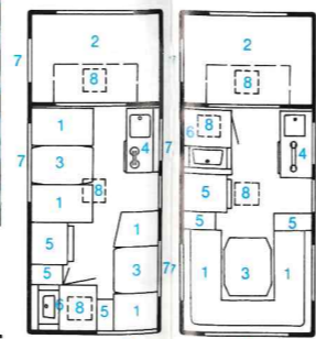
Zeichenerklärung: 1 = Sitzbank 2 = Stationäres Bett 3 = Tisch 4 = Küche 5 = Schrank 6 = Toilettenraum 7 = Ausstellfenster 8 = Dachhaube
